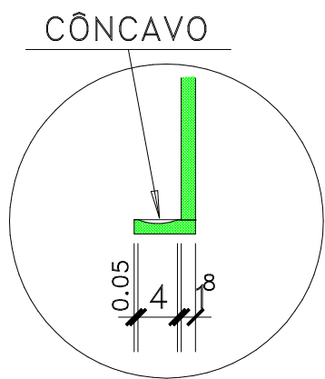
Detalhe: -Ampliado
