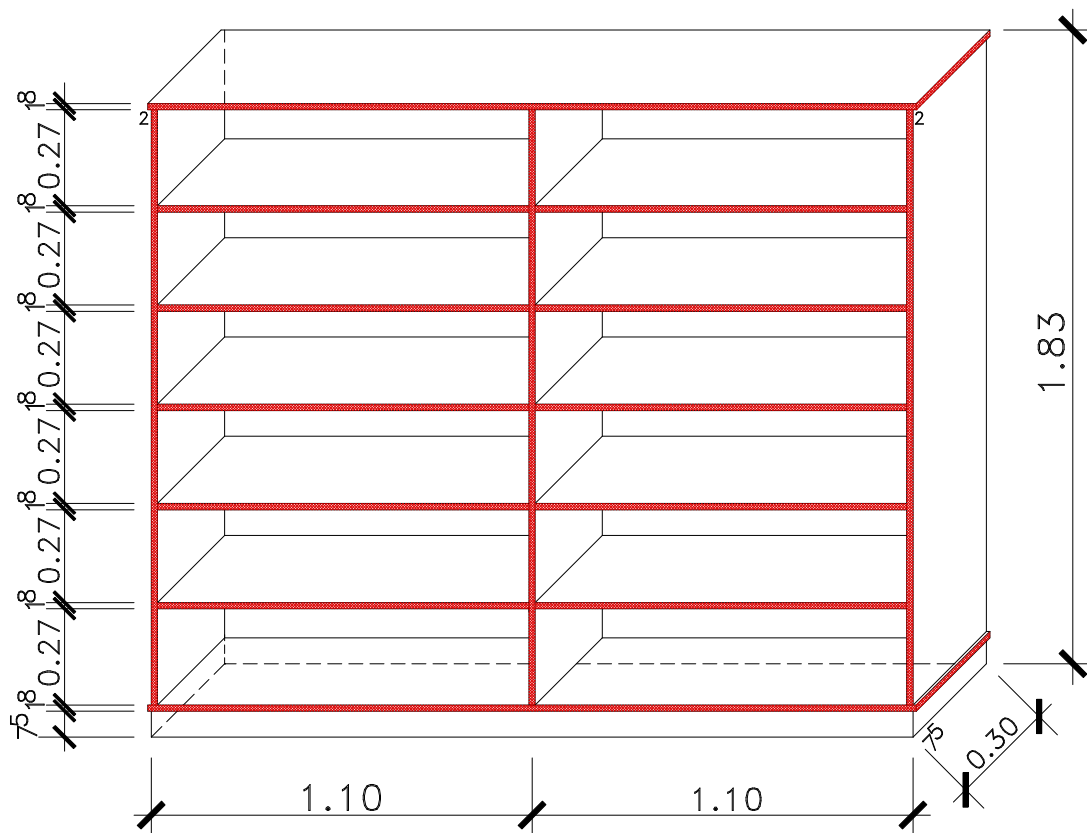
PERSPECTIVA
