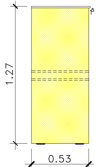
Vista Lateral
